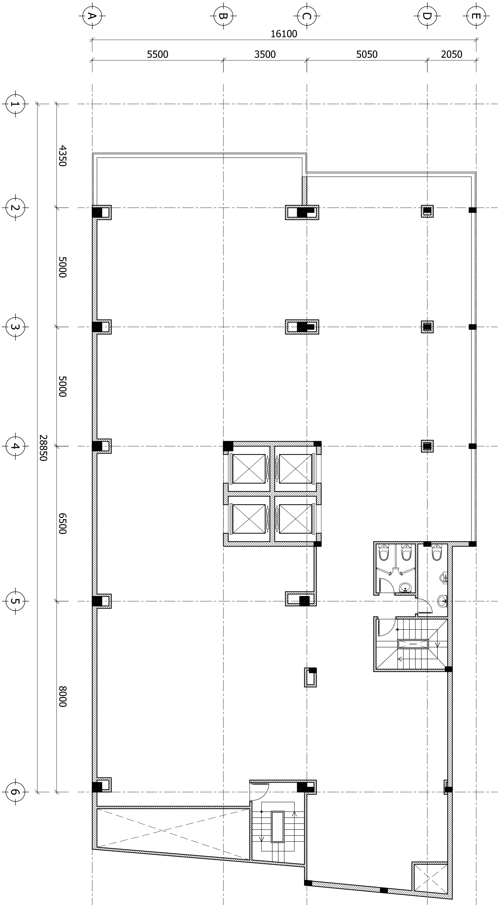
MẶT BẰNG TẦNG 1-11 TỈ LỆ :1/100 (PHÂN KHU)
